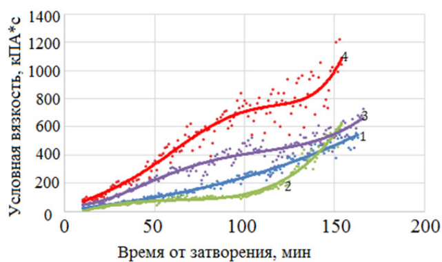
Рис. 2. Диаграммы кинетики схватывания цементного теста: концентрация НЦ: 1 – без НЦ; 2 – 2,4 \cdot 10^{-4} ; 3 – 2,4 \cdot 10^{-3} ; 4 – 2,4 \cdot 10^{-2}
