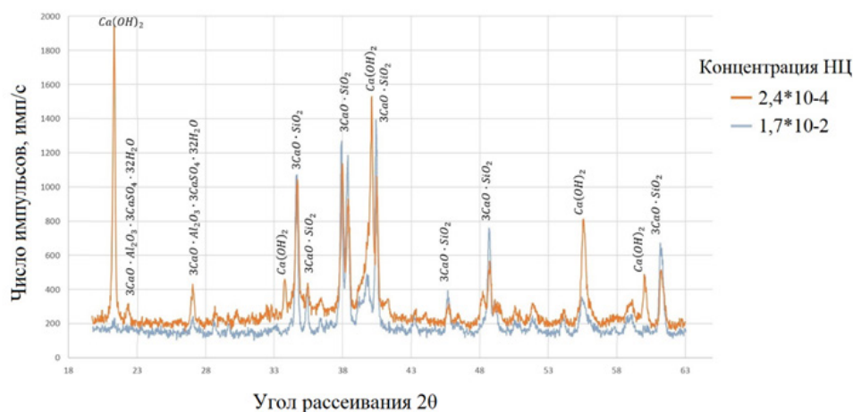
Рис. 5. Влияние nanoцеллюлозы на фазовый состав цементного композита
