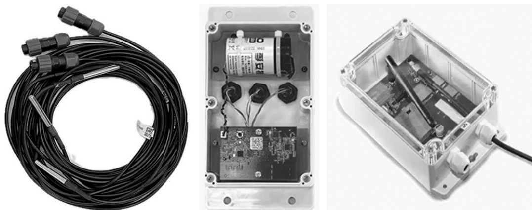
Рис. 1. Комплект системы термомониторинга (слева направо: датчики температуры, термолоттер, сетевой шлюз)
